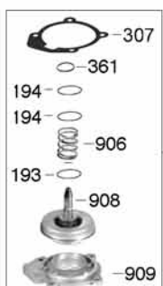
Servo
